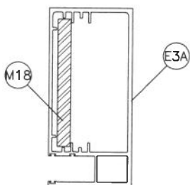
JAMB 'J3'
